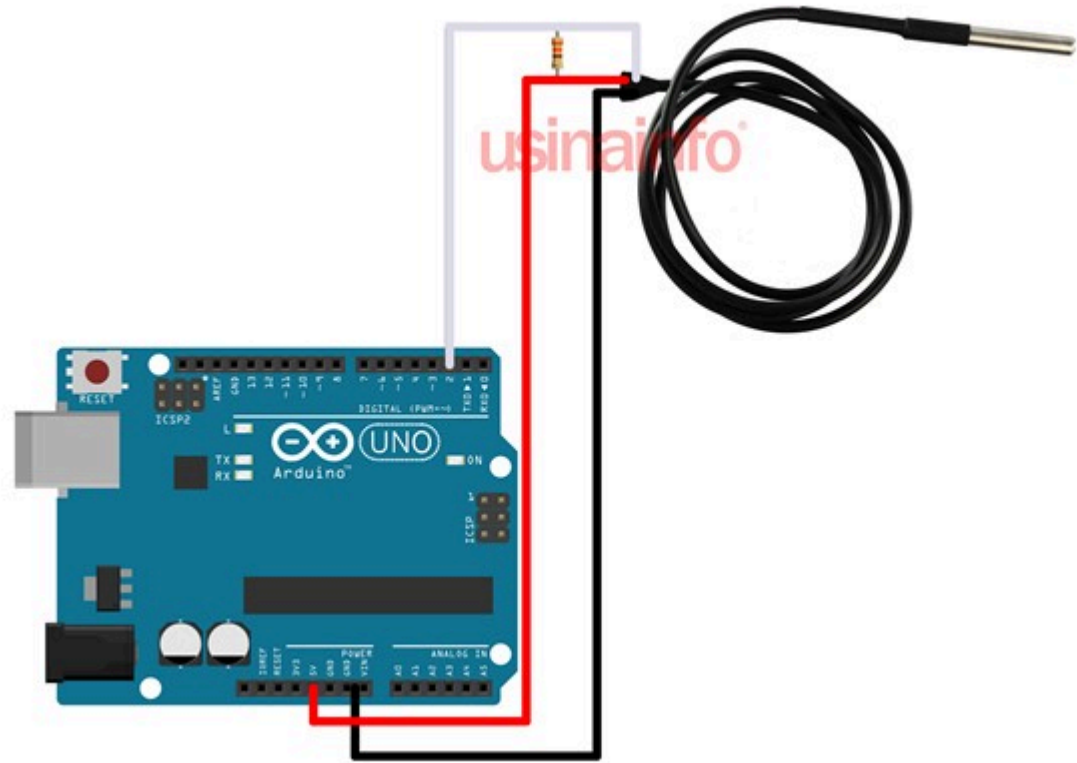
Sensor de Temperatura DS18B20 com Arduino
